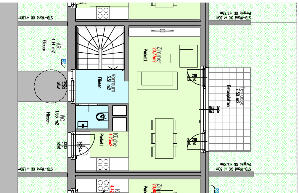
GRUNDRISS ERDGESCHOSS
